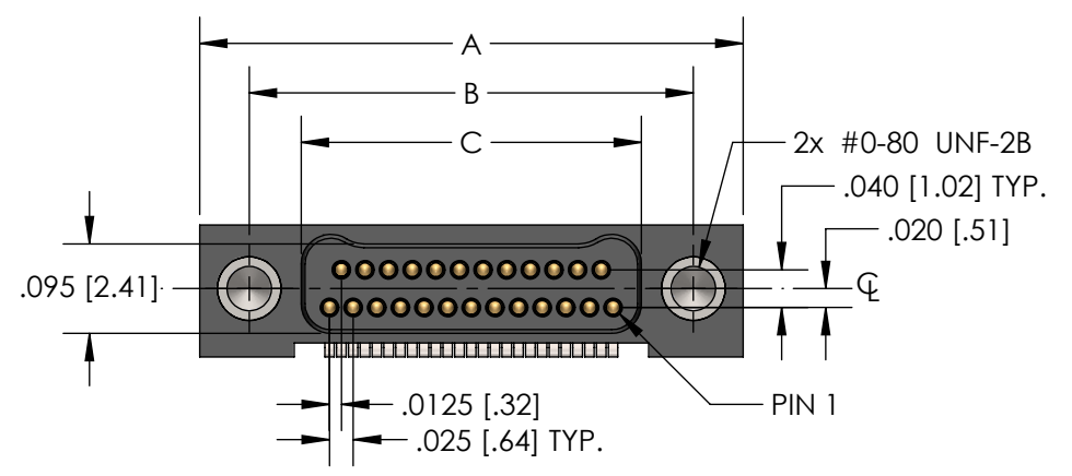
PLUG (PINS)
