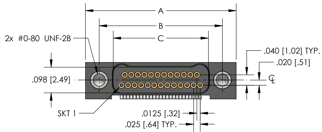
RECEPTACLE (SOCKETS)
